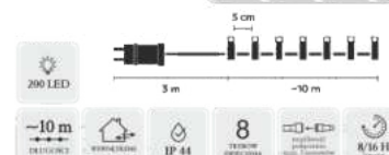
LAMPKI LED 200L ZIMNY BIAŁY DŁ. 3 + 10 M WERN/ZERN
