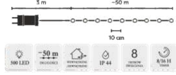
LAMPKI LED DRUCIKI NA SZPULI 500L ZIMNY BIAŁY, DŁ. 3 + 50 M
