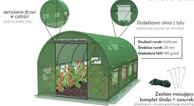
TUNEL FOLIOWY OGRODOWY 4 SEGMENTOWY ZIELONY NEW SOLUTION 4 x 2,5 x 2 M
