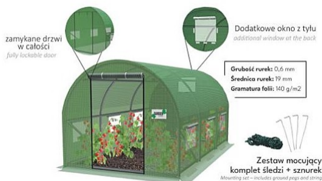
TUNEL FOLIOWY OGRODOWY 3 SEGMENTOWY ZIELONY NEW SOLUTION 3 x 2 x 2 M
