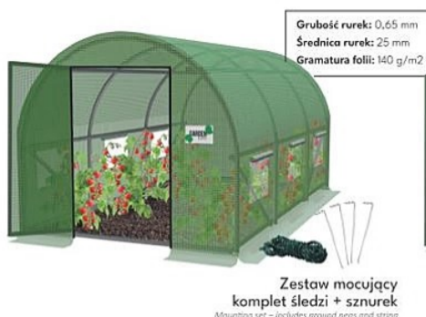
TUNEL FOLIOWY OGRODOWY 3 SEGMENTOWY ZIELONY 4 x 2,5 x 2 M Z DRZWIAMI NA ZAWIASIE
